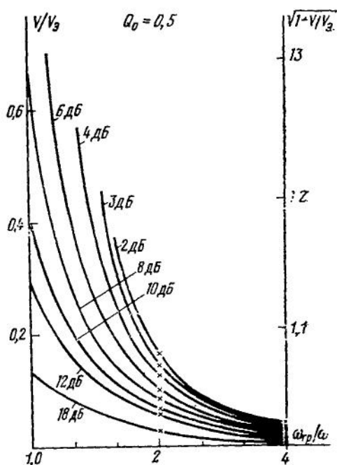
РИС. 42. Зависимость V_a/V от \omega_{gp}/\omega_0 при Q=0,5
