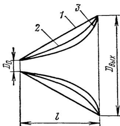
РИС. 70. Профили применяемых рупоров
