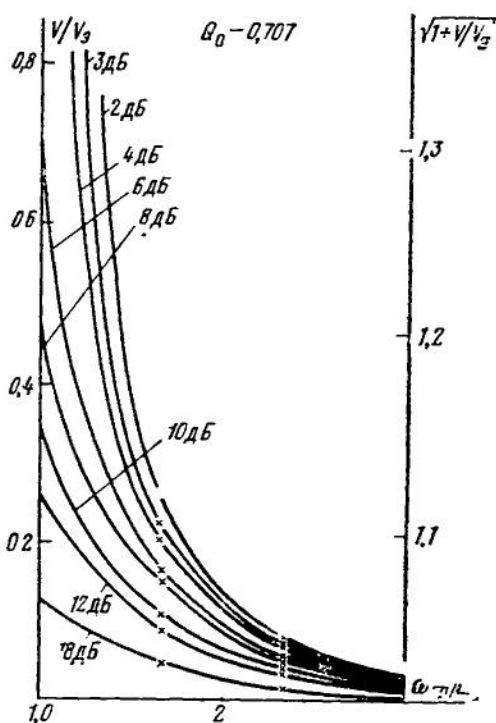
РИС. 44. Зависимость V_a/V от \omega_{gp}/\omega_0 при Q=0,7
