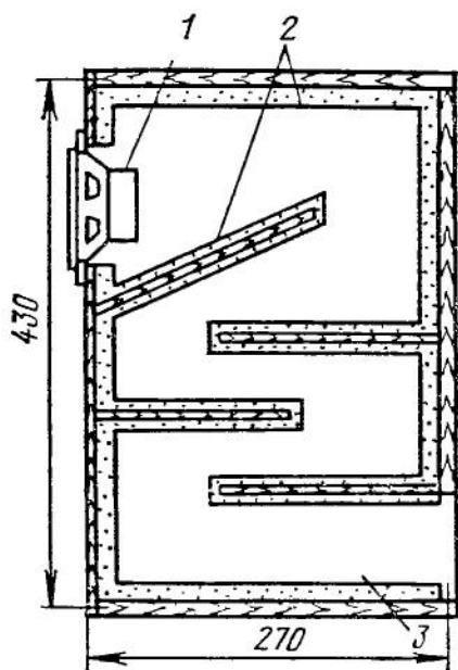
РИС. 68. Лабиринт фирмы Akai в разрезе
