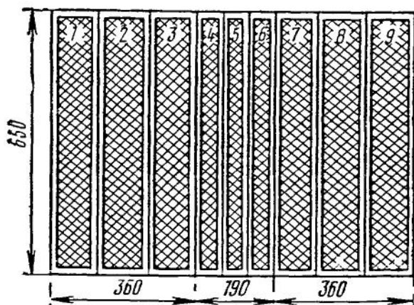
РИС. 74. Изображение широкополосной электростатической акустической системы ГСП-1
