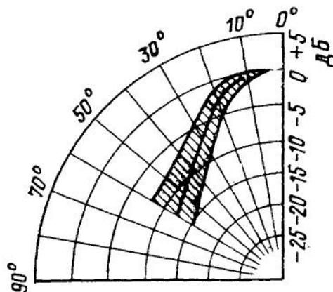
РИС. 87. Зависимость коэффициента использования площади прослушивания от направленности громкоговорителей для разных углов пере-сечения акустических осей
