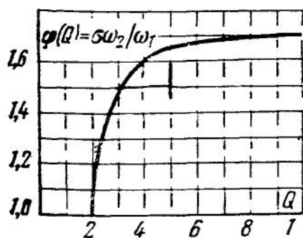
РИС. 31. Зависимость \varphi(Q) от Q
