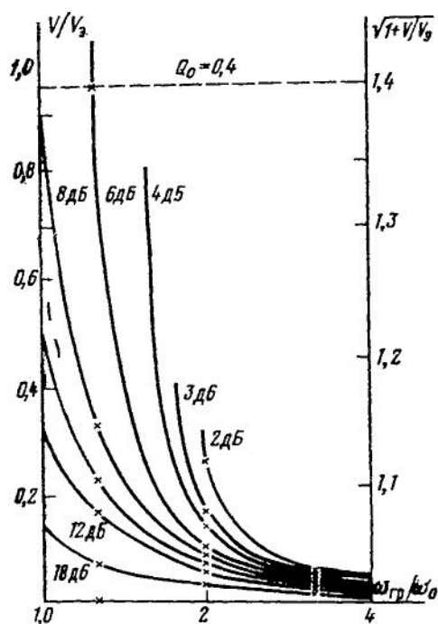
РИС. 41. Зависимость V_a/V от \omega_{gp}/\omega_0 при Q=0,4
