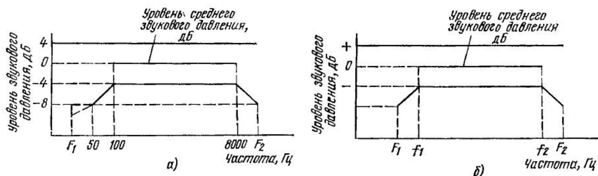
РИС. 16. Поля допусков частотной характеристики звукового давления АС: а — высшей (0) группы сложности; б — 1, 2 и 3 групп сложности
