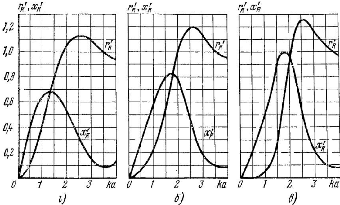
РИС. 10. Удельное сопротивление излучения различных видов излучателей
