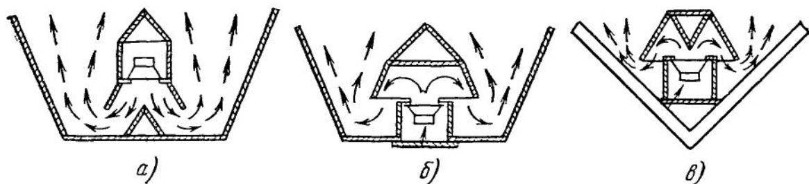
РИС. 73. Конструкции свернутых рупоров
