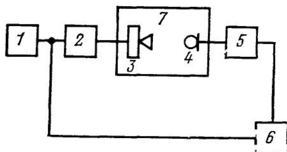
РИС. 92. Схема измерения частотных характеристик
