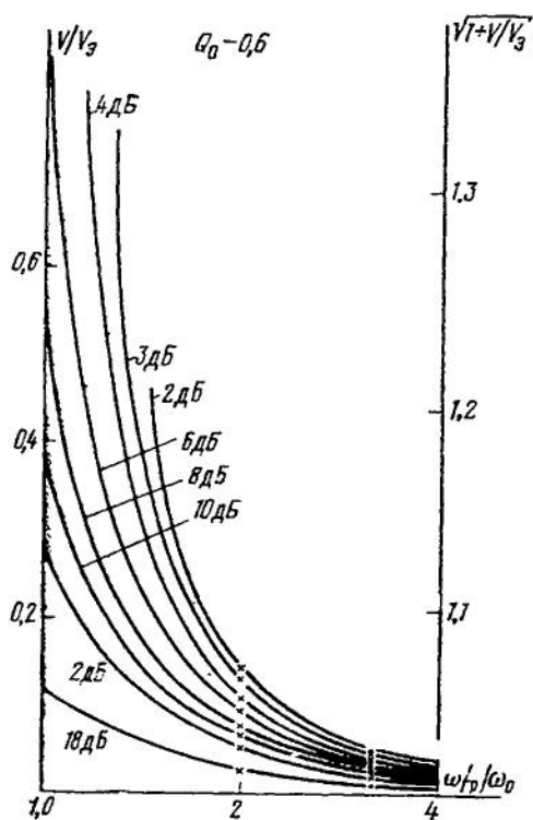
РИС. 43. Зависимость V_a/V от \omega_{gp}/\omega_0 при Q=0,6
