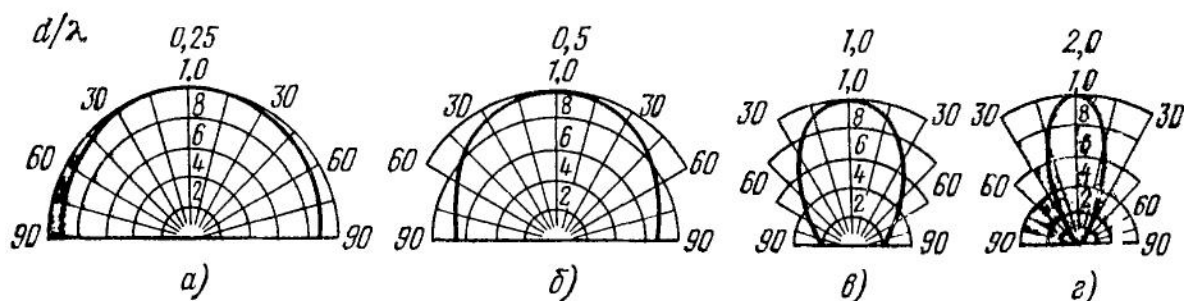
РИС. 13. Характеристики направленности излучения поршня в бесконечном экране при различных отношениях d/\lambda .
